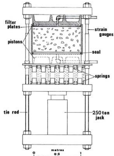
(b) Floating ring (Penman et al, 1976)
